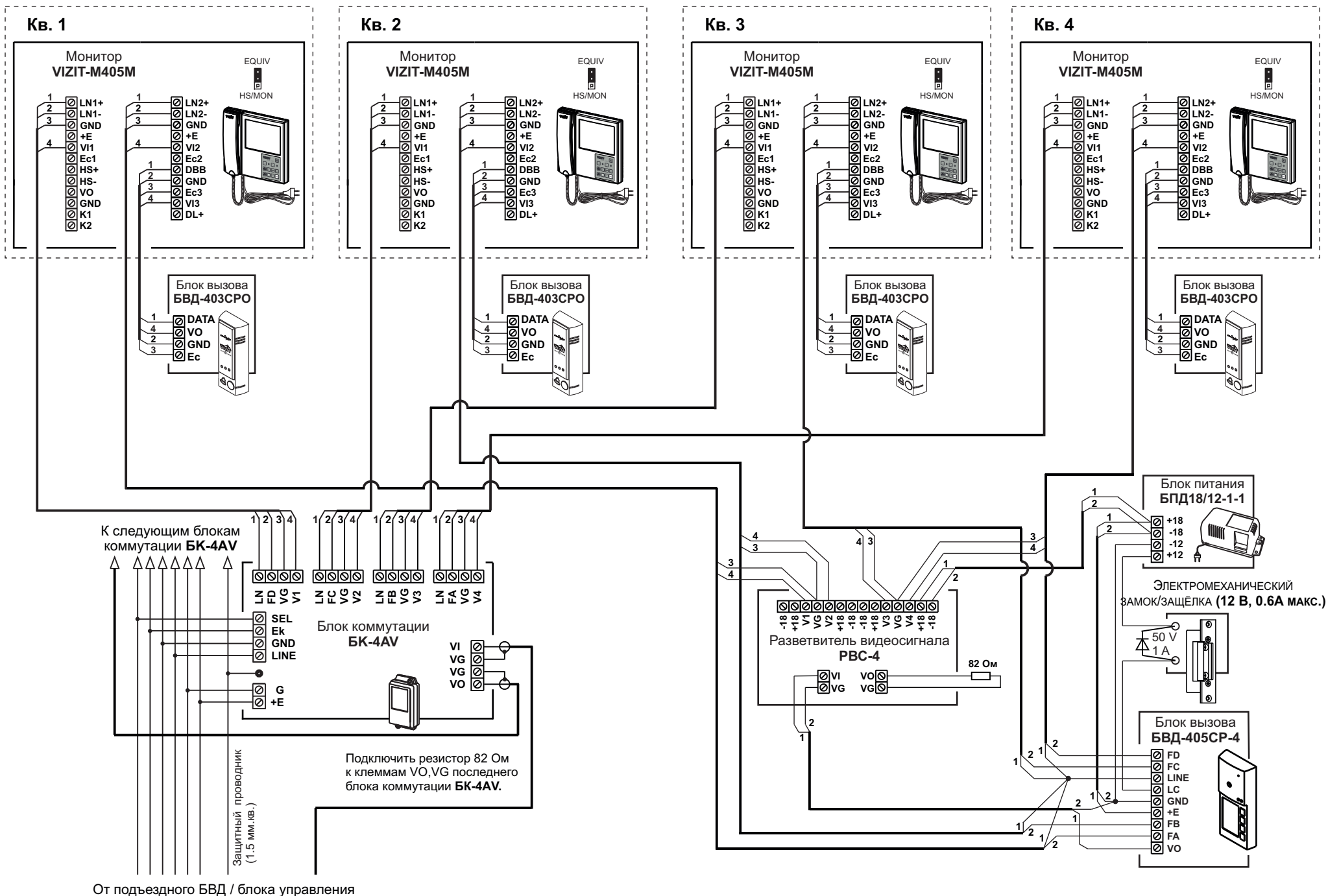
Рисунок 10 - Схема соединений мониторов VIZIT-M405M с блоком коммутации БК-4АВ и блоком вызова БВД-405СР-4
